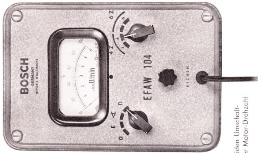
Linker Umschaltknopf auf Stellung "n" (Drehzahl)
